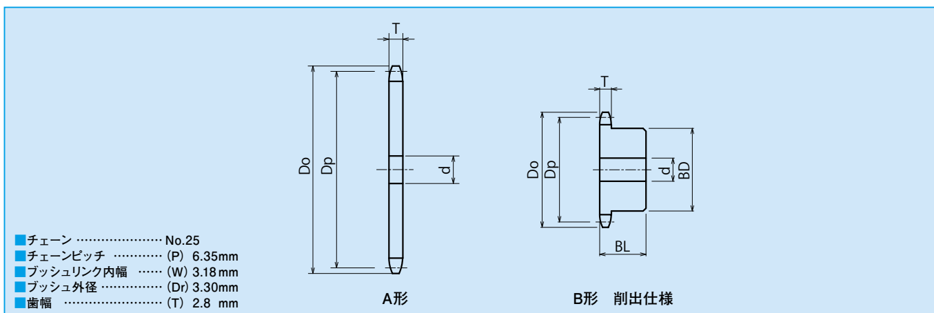
○寸法表
